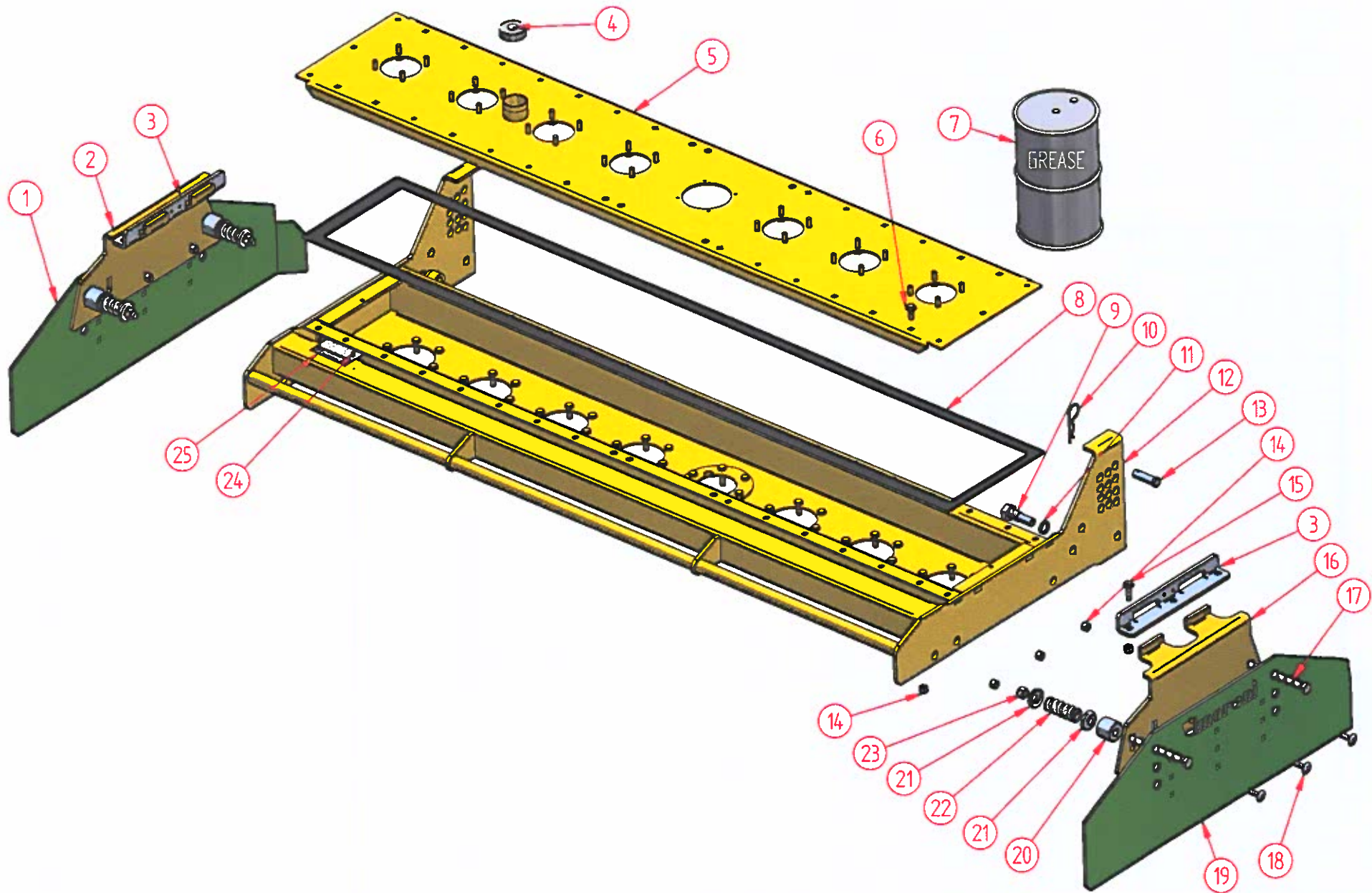
CASSAFORMA ERPICI FISSI - POWER HARROWS CASE
