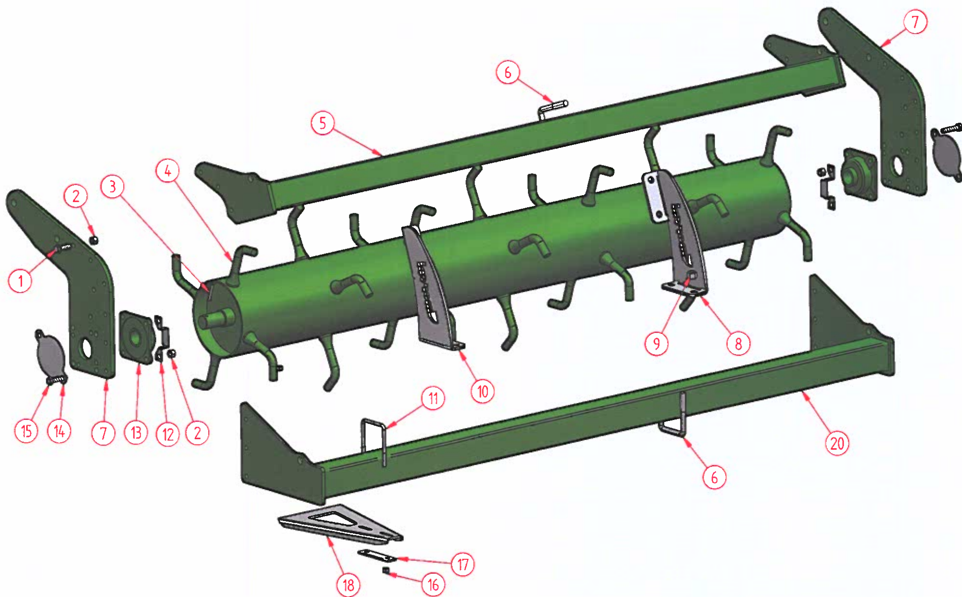
RULLO SPUNTONI - SPIDEK ROLLER
