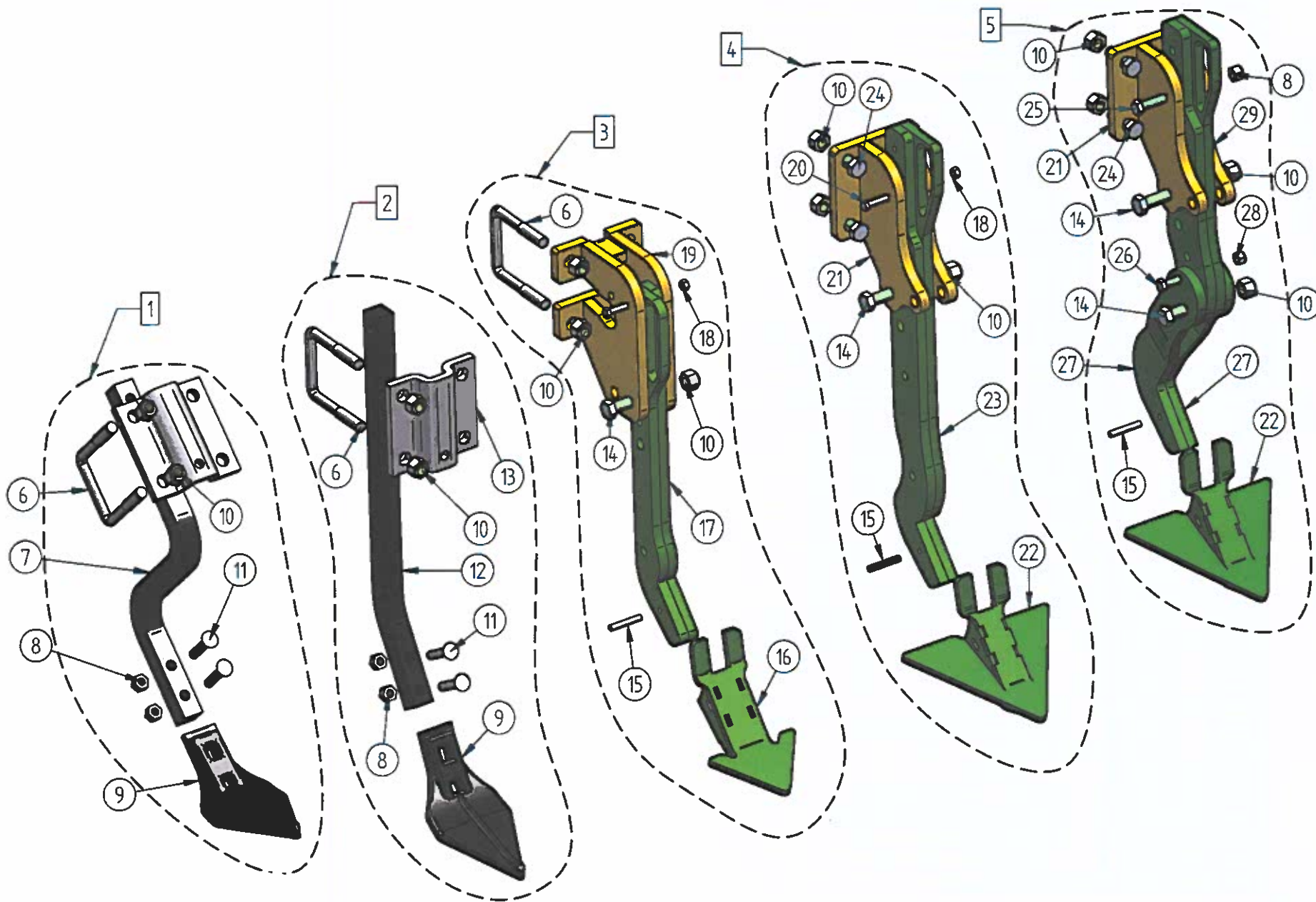
ROMPITRACCIA ERPICI - WHEEL MARK ERADICATOR
