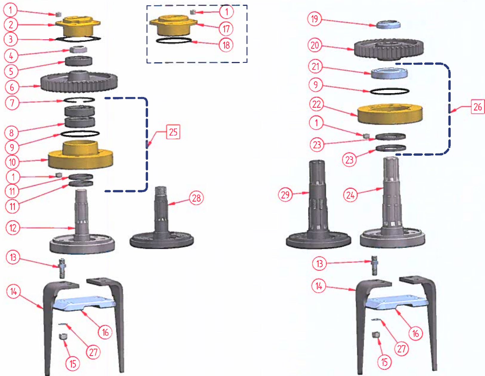
MOVIMENTAZIONE KRONOS - KRONOS ROTORS
