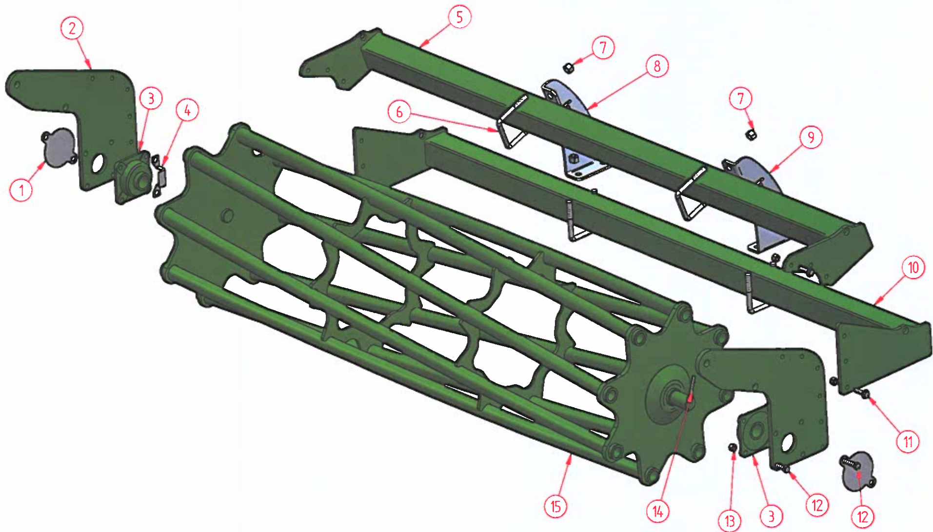
RULLO GABBIA Ø540 - CAGE ROLLER Ø540
