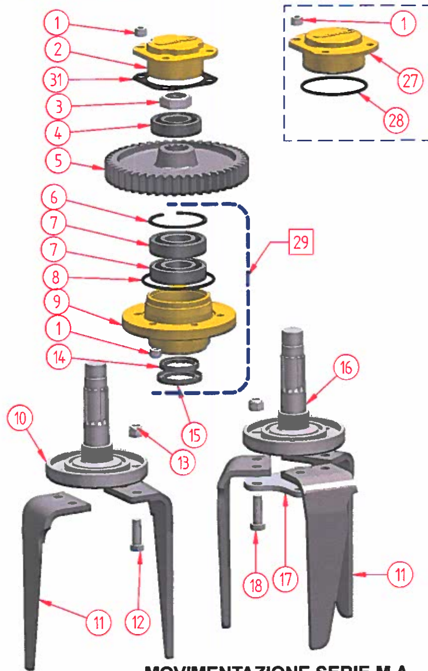
MOVIMENTAZIONE SERIE M.A. - SERIE M.A. ROTORS
