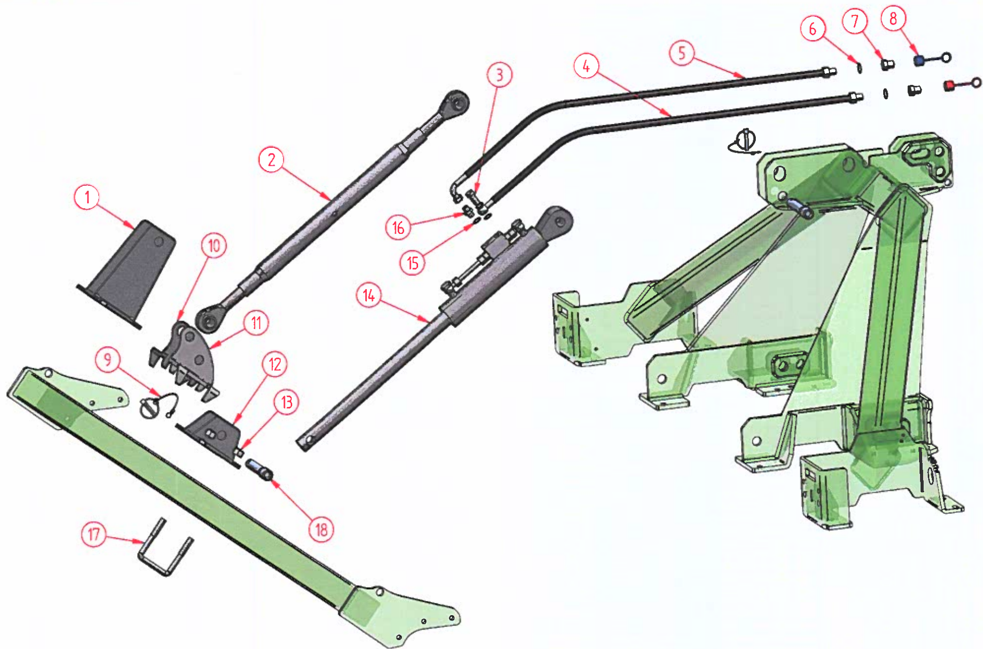
REGISTRO RULLO IDRAULICO FISSO - HYDRAULIC ADJUSTABLE ROLLER
